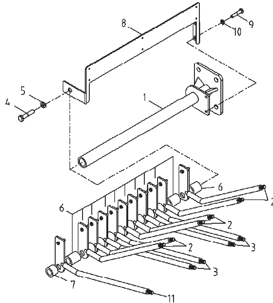
레버 스탠드 셋 Fig. 3-2-2 SCS1616 LEVER STAND SET
