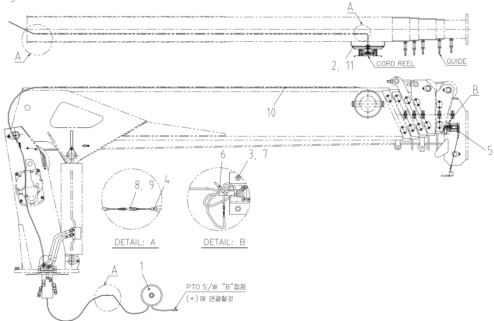
Fig. 15 과권방지장치 조립체
