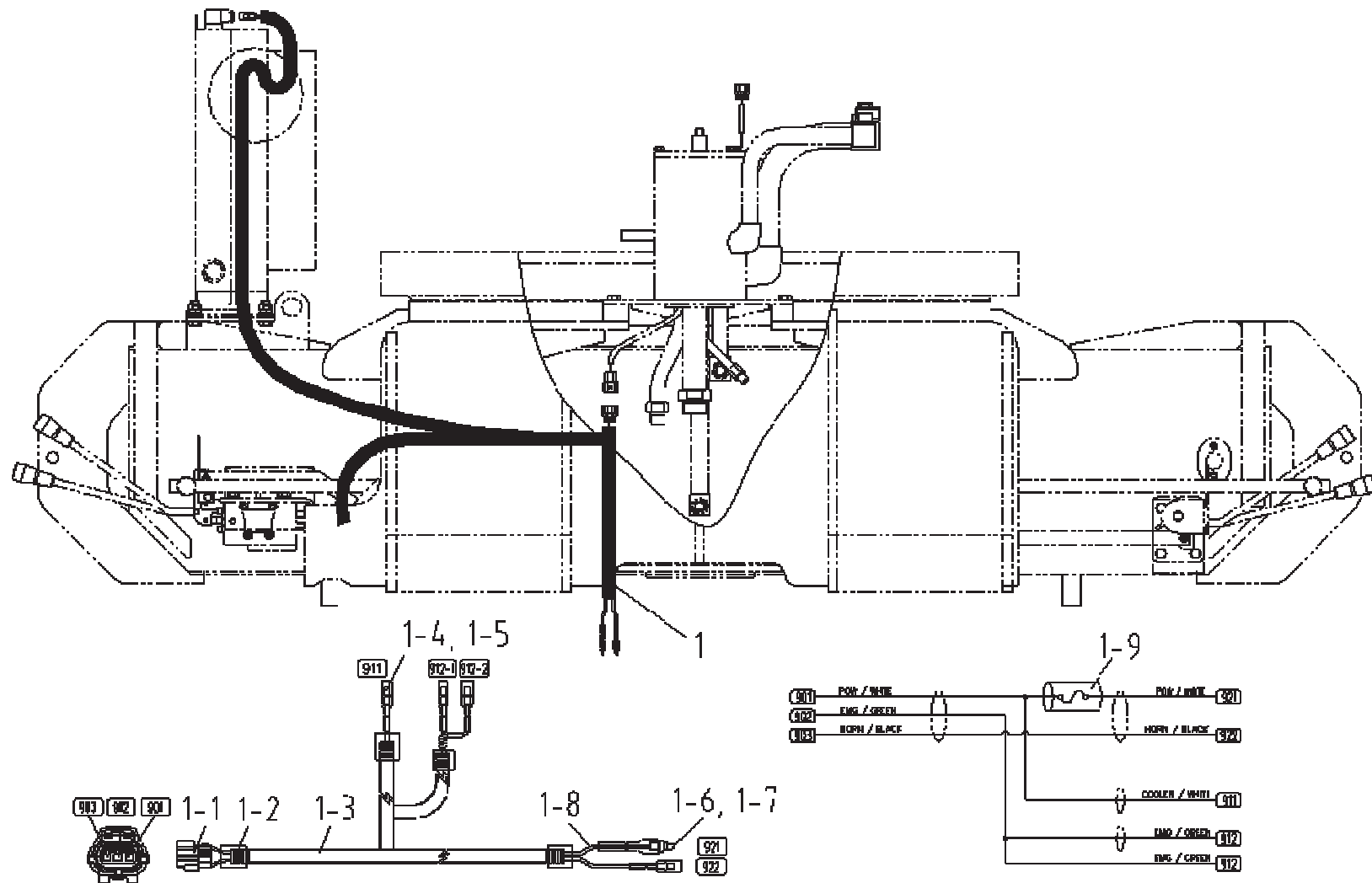
프레임 전선 Fig. 10-1 SCS1616 FRAME WIRING
