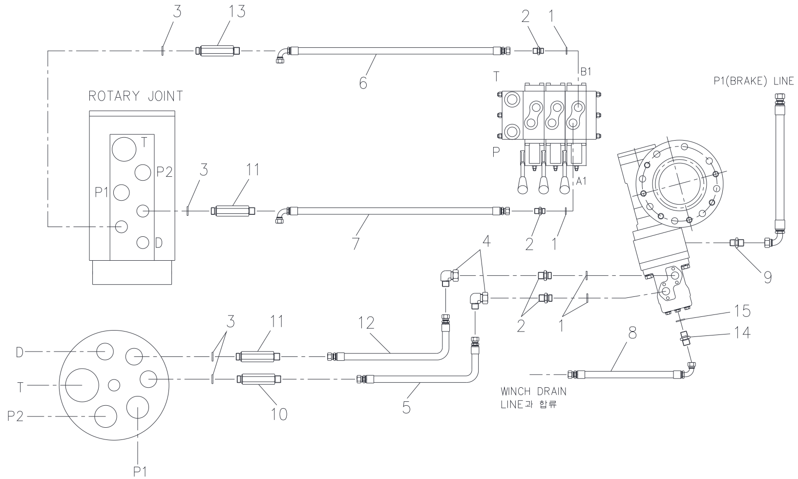
스윙 배관 Fig. 5-2 SCS1616 SWING PIPING
