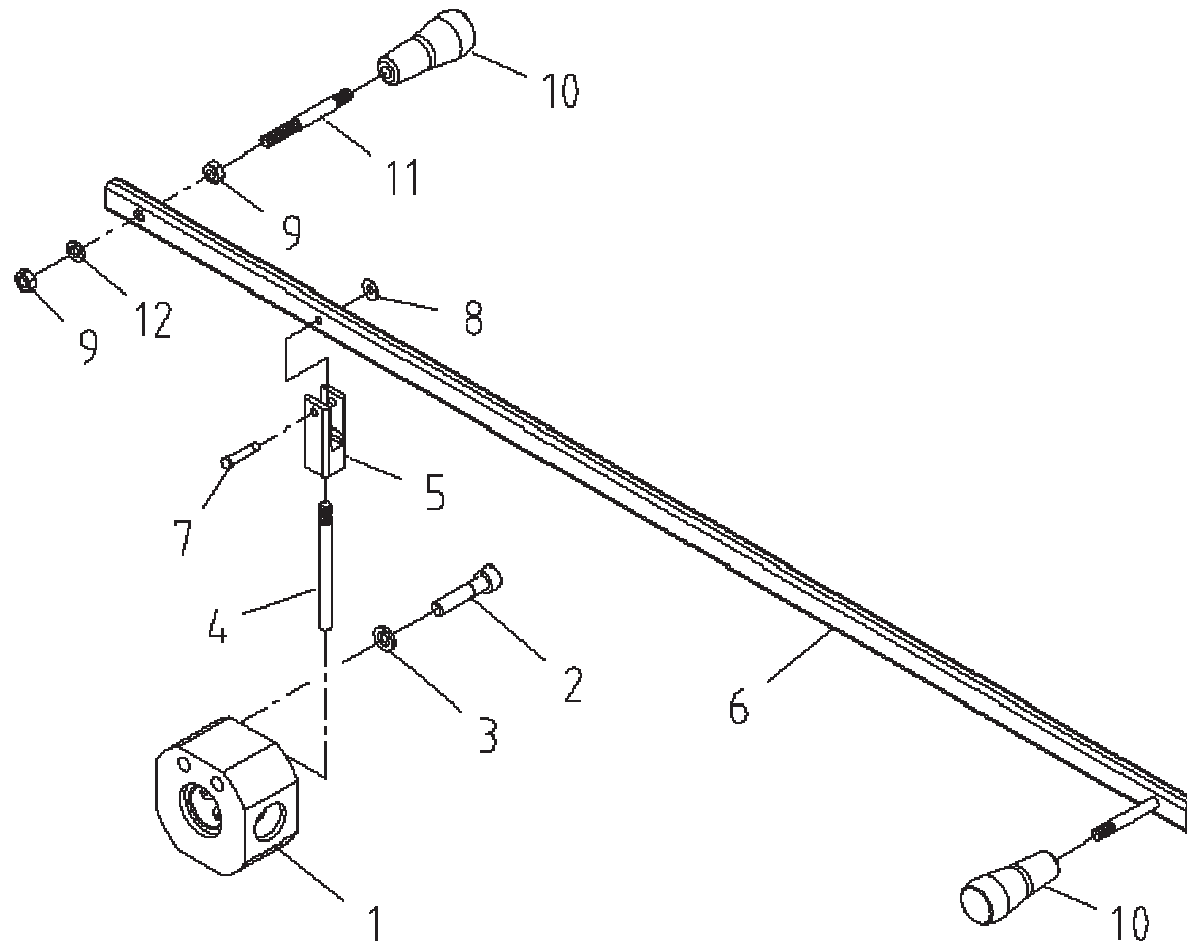
디버터 밸브 셋 Fig. 3-1 SCS1616 DIVERTER V/V SET
