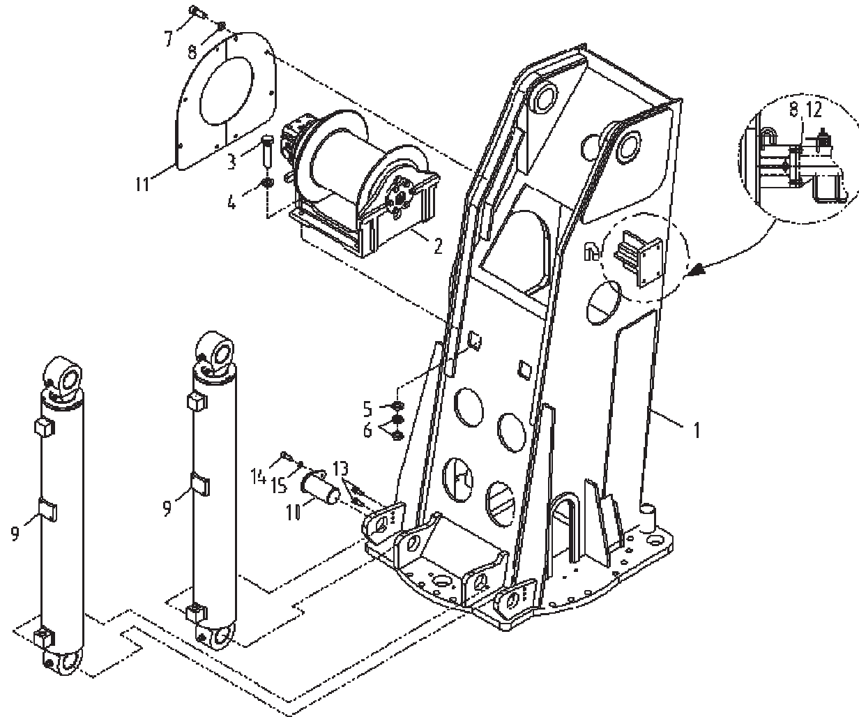
스윙 포스트 조립체 Fig. 2 SCS1616 SWING POST ASS'Y
